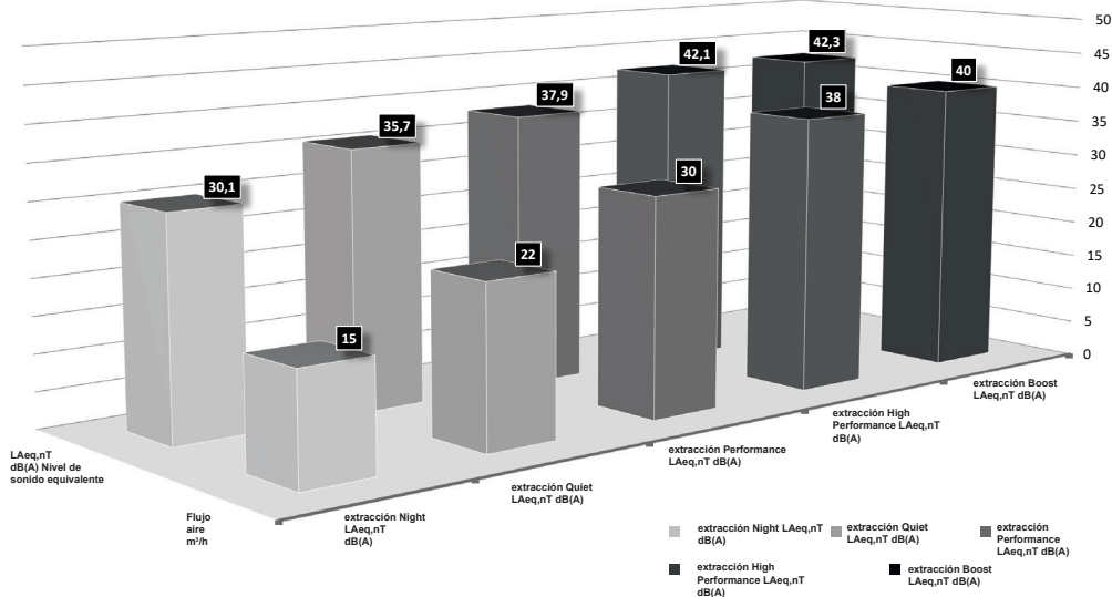
VORT HRW 40 MONO EVO WiFi - Gráfico Flujo aire / Nivel de presión de sonido continuo equivalente (extracción)
